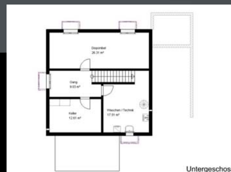
Untergeschoss
